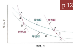
図 3A-7 カルノーサイクルの基本構造。段階1は温度 T_h における可逆な等温膨張である。段階2は可逆な断熱膨張で、温度は T_h から T_c に低下する。段階3は T_c における可逆な等温圧縮で、つづいて起こる可逆な断熱圧縮で系は始状態に戻る。
