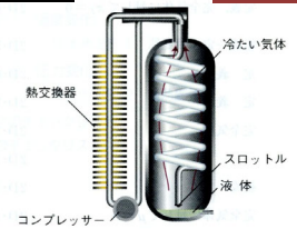
図 2D-12 リンデの冷凍機の原理を示す図。気体を冷却させるので、その温度が上部逆転温度以下にある限り、スロットルを通して膨張すれば冷却が起こる。冷却された気体が高压側の気体を冷やし、その冷えた気体がさらに膨張で冷却する。ついには液化した気体がスロットルから滴下する。
