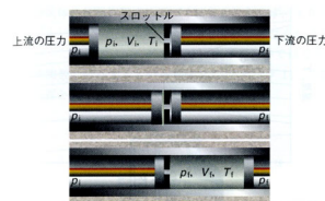
図 2D-7 ジュール・トムソンの膨張の熱力学的基礎を説明する図。ピストンは上流と下流の気体を表し、これがスロットルの両側でそれぞれ一定の圧力を維持する。上の図から下の図へいくにつれて、一定量の気体がスロットルを通過する様子を示す、それがエンタルピーの変化なしに起こる。
