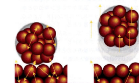
図 3A-2 第二法則が表す非可逆性の分子論的解釈。(a) 温かい表面上に静止しているボール。原子は矢印で示したように熱運動(この例では振動)している。(b) ボールが上方
