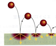
図 3A-1 床の上で弾んでいるボールに起こる自然な変化の向き。弾むごとにそのエネルギーのいくぶんかが床の構成原子の熱運動へと劣化し、散逸していく。その逆が巨視的なスケールで起こることは、まず観測されない。
