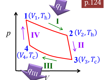
図 3A-8 エネルギー q_1 (たとえば 20 kJ) が熱機関に供給され、 q_2 (たとえば、 q_2 = -15 kJ) が熱機関から失われて低温シリンダに捨てられるとする。熱機関によってなされる仕事は |q_1| - |q_2| (たとえば、20 kJ - 15 kJ = 5 kJ) となる。効率は、高温熱源から得られた熱で、なされた仕事を除いたものである。
