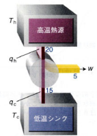
図 3A-8 エネルギー q_1 (たとえば 20 kJ) が熱機関に供給され、 q_2 (たとえば、 q_2 = -15 kJ) が熱機関から失われて低温シリンダに捨てられるとする。熱機関によってなされる仕事は |q_1| - |q_2| (たとえば、20 kJ - 15 kJ = 5 kJ) となる。効率は、高温熱源から得られた熱で、なされた仕事を除いたものである。
