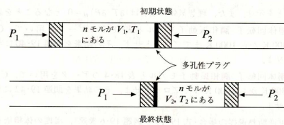
図 19-11 ジュール・トムソンの実験の概略図。
