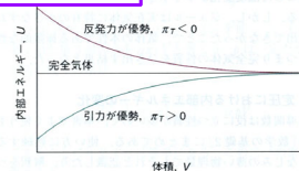
図2D・4 完全気体では、内部エネルギーは(一定温度では)体積に依存しない。実在気体で引力が優勢な場合、体積が増加すると、分子は平均としていっそう離れることになるから内部エネルギーは増加する。反発力が優勢な場合、内部エネルギーは気体の膨張によって減少する。
