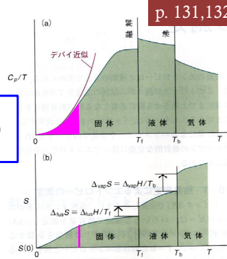
図 3B-1 熱容量データからのエントロピーの計算。(a) ある試料の C_p/T の温度変化。(b) エントロピーの温度変化。ある温度 T におけるエントロピー S(T) は、0 K から温度 T までの (a) の曲線 C_p(T)/T の下の部分の面積に、途中にある相転移それぞれのエントロピー \Delta_{\text{trs}}S を加えたものに等しくなる。
