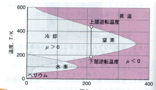
図 2D-11 3種の実在気体、窒素、水素、ヘリウムの逆転温度。
