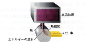
図 3A-3 第二法則のKelvinの表現は、ここに描かれた、熱が完全に仕事に変換され、それ以外には何の変化も残さないような過程の可能性を否定する。この過程ではエネルギーは保存されているので第一法則とは矛盾しない。
