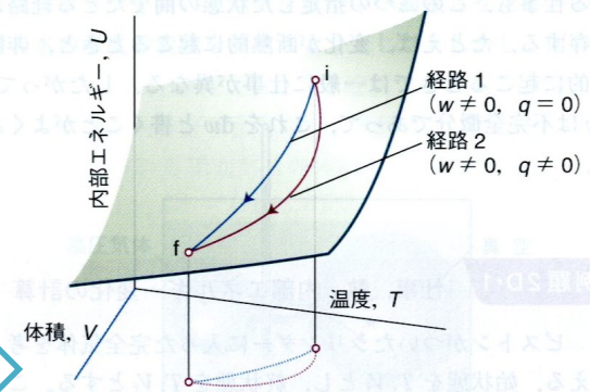
図 2D-1 系の体積と温度が変わると内部エネルギーが変化する。図の経路 1 と経路 2 はそれぞれ断熱経路と非断熱経路を表す。この二つでは q と w は異なる値であるが、 \Delta U の値は同じである。
